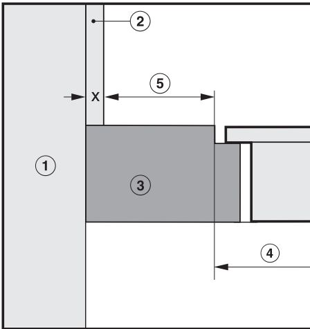
완전 매립형 쿡탑
