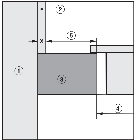
준매립형 쿡탑
